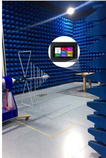
图 3-5 辐射测试图
