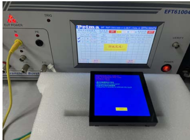
图 3-4 群脉冲测试图
