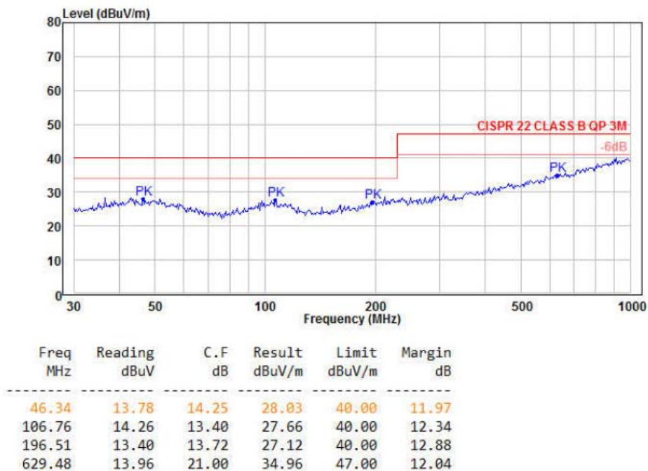
图 3-7 辐射测试垂直方向
