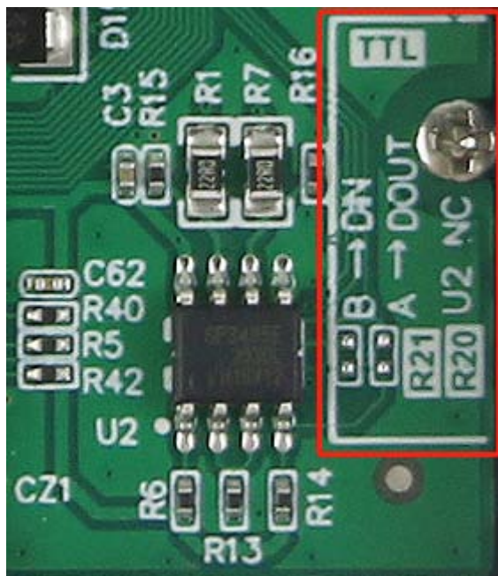
图 6-1RS485 和 TTL 转换电路
