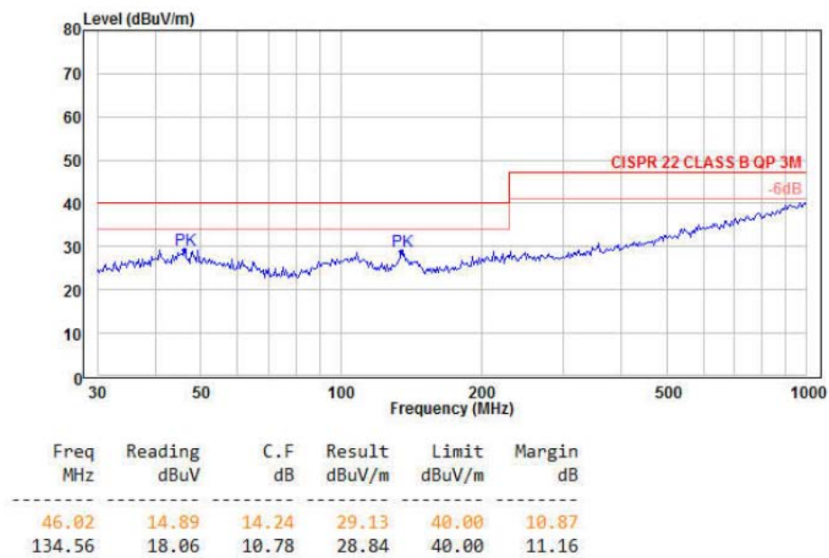
图 3-6 辐射测试水平方向
