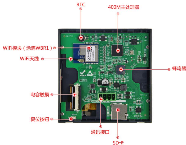
图 1-2 硬件配置图
